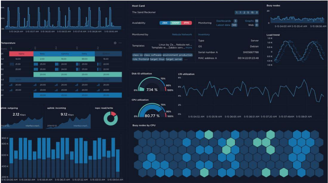
Zabbix UI
